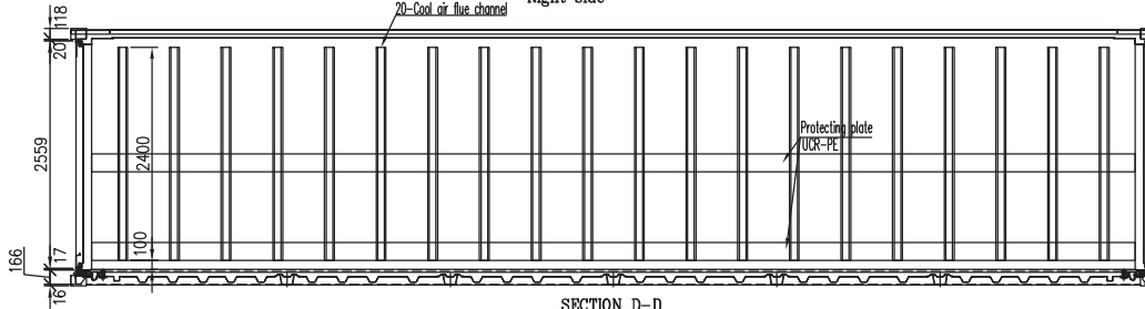
SECTION D-D
